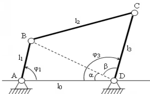
Рис.1. Расчетная схема МПС.
