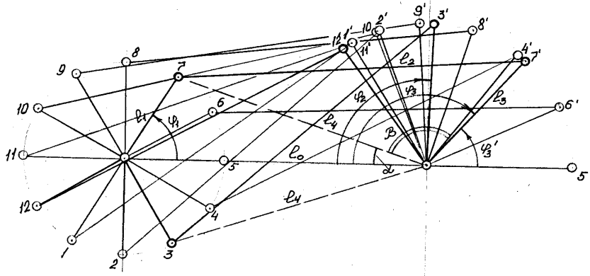
Рис.2. Схема положений ударного МПС.
