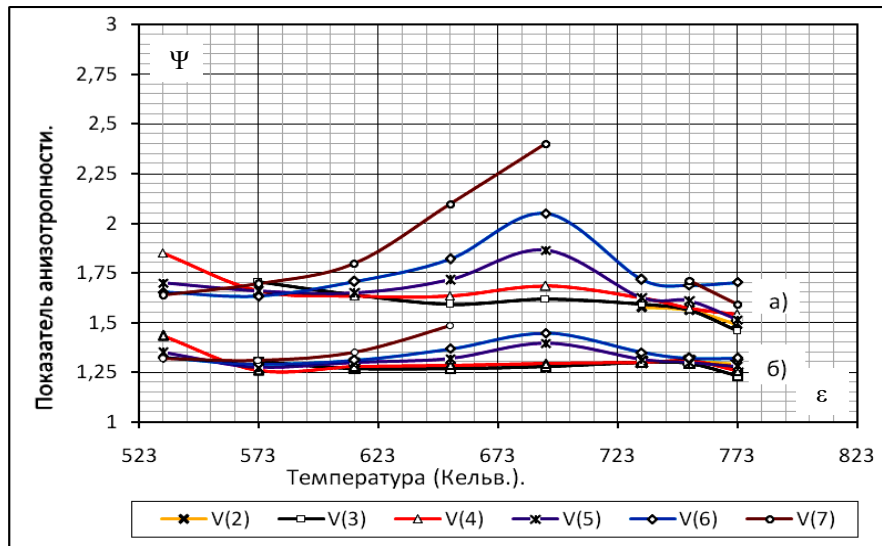
Рис. 1. Изменение показателя анизотропности ( \Psi ) от температуры ( \theta ) при скоростях деформирования:
