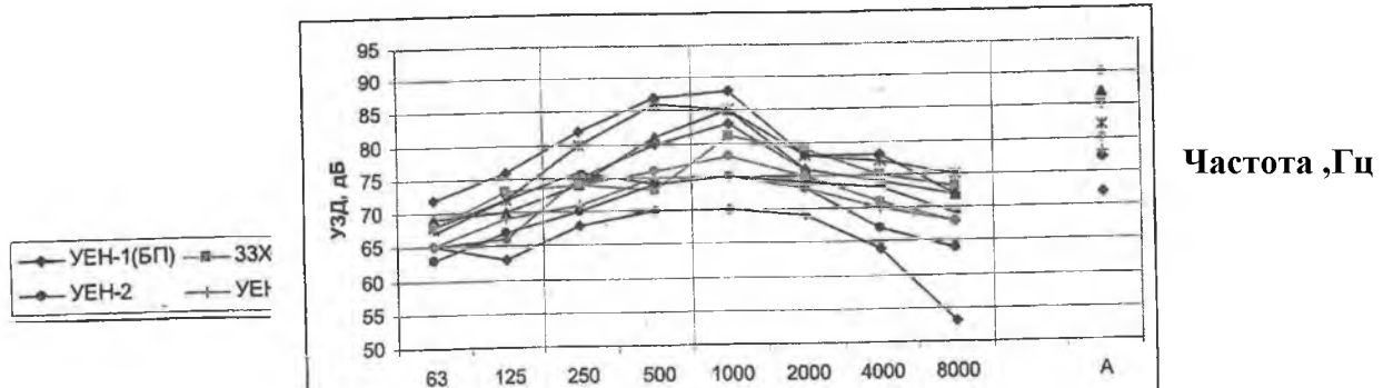
Рис.3. Уровни звука
